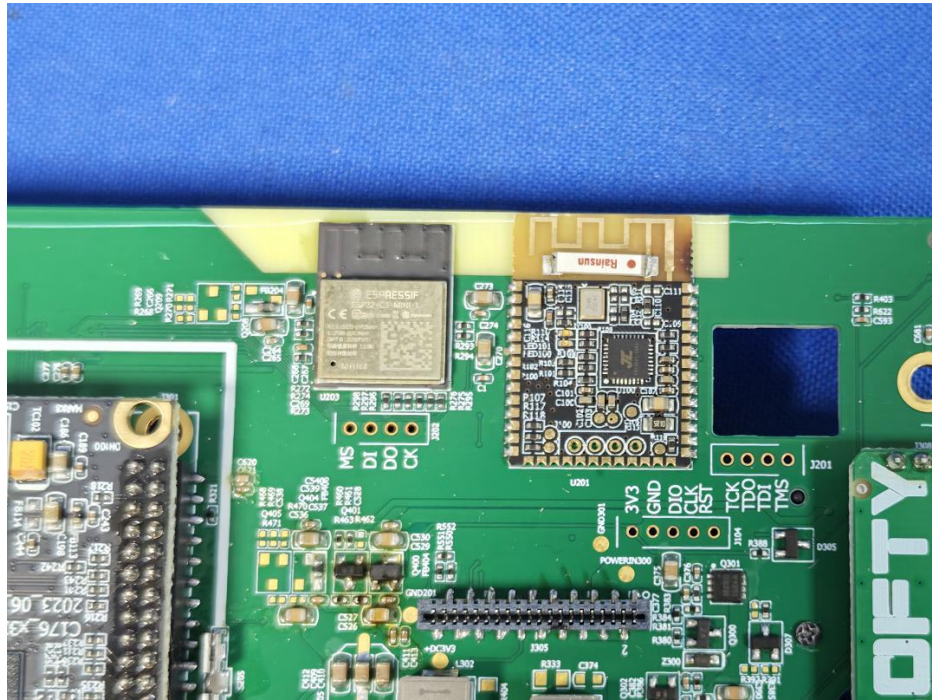
BT ANT
