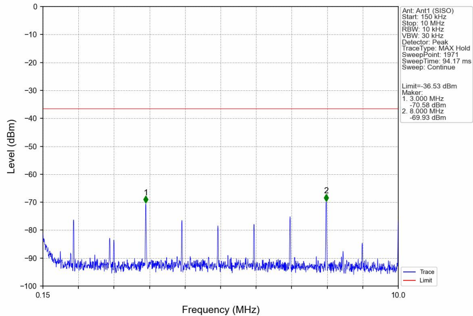
802.11b_LCH_2412MHz_Ant1 (SISO)_NTNV
