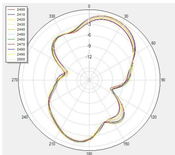
V Phi=0
