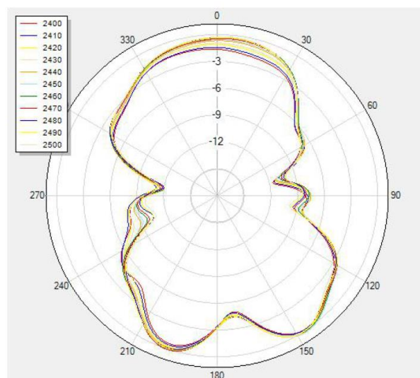
V Phi=90
