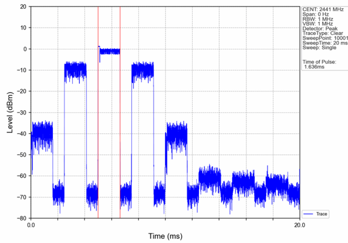
Pi/4DQPSK_2DH3_HOPP_Ant1_NTNV
