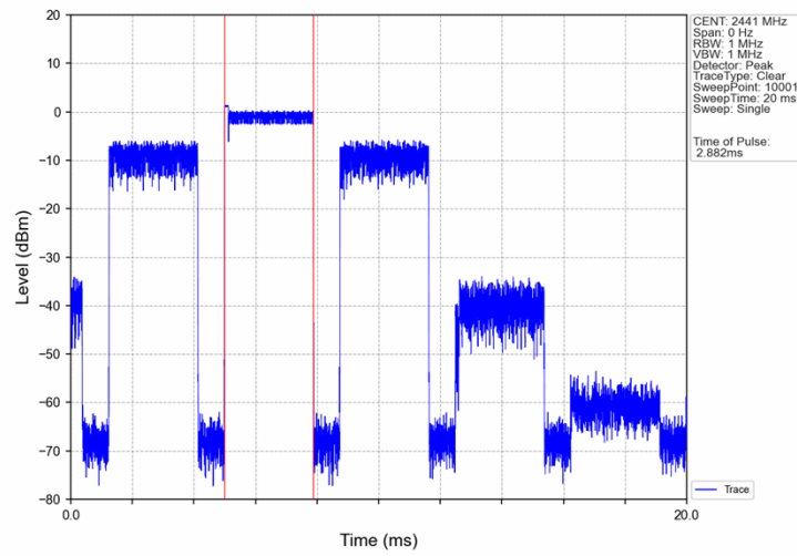
Pi/4DQPSK_2DH5_HOPP_Ant1_NTNV
