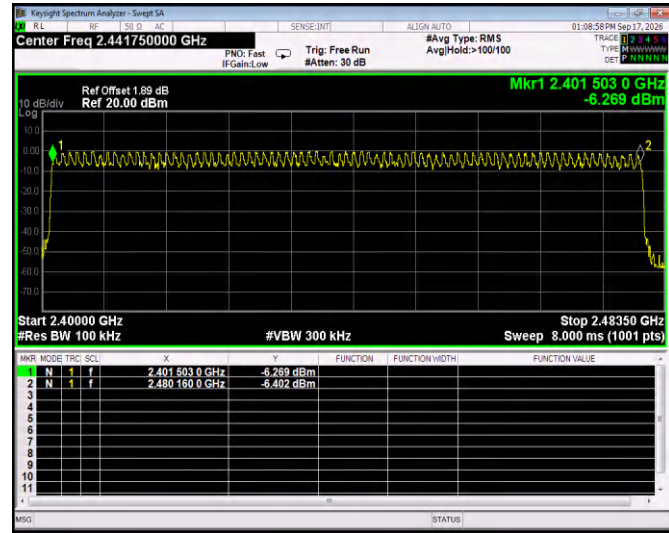
\pi/4 -DQPSK - 2-DH1 Test Plots
