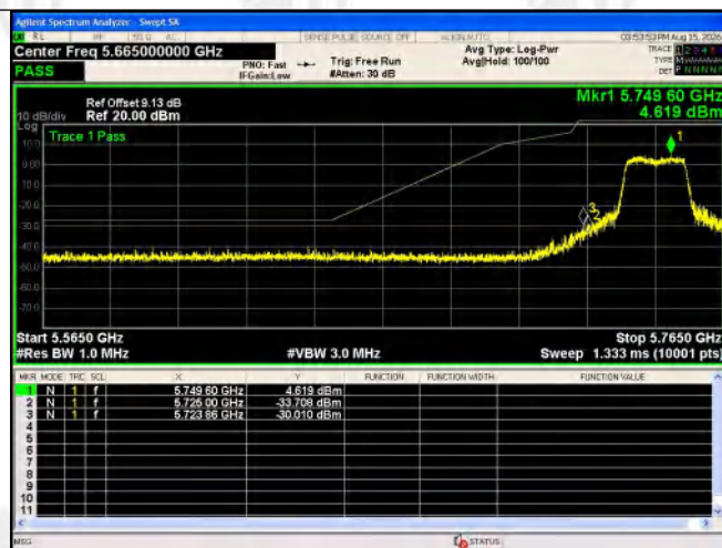
802.11(n40)-5755
