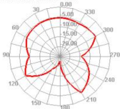
2400.000MHz E2
