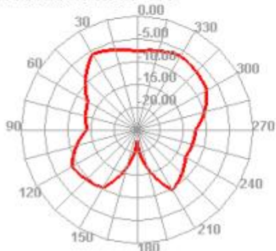
2400.000MHz E1
