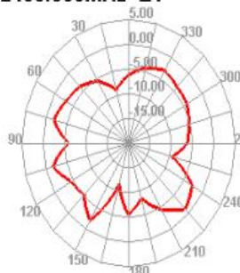
2400.000MHz E1
