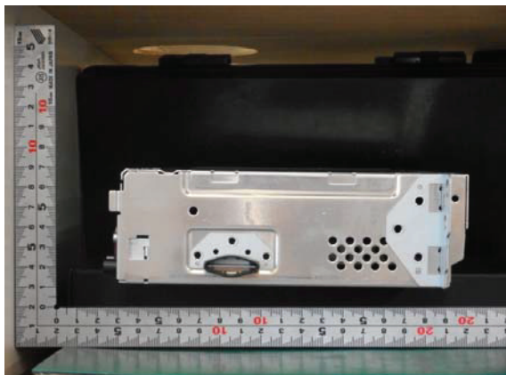
LEFT Veiw
