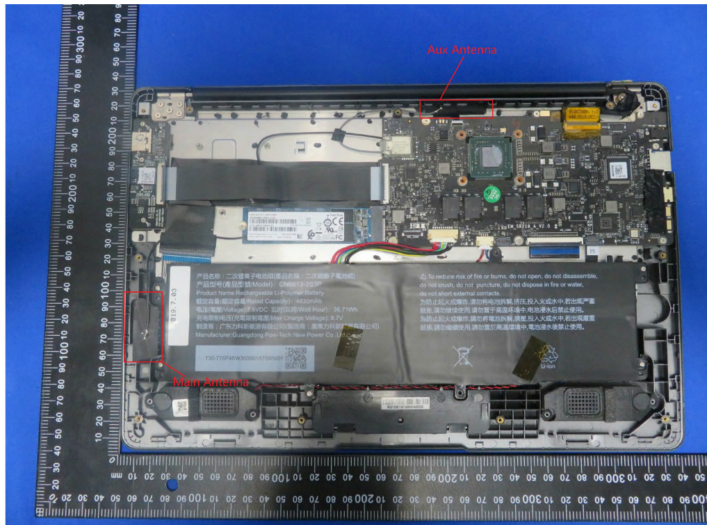
(2) EUT Photo
