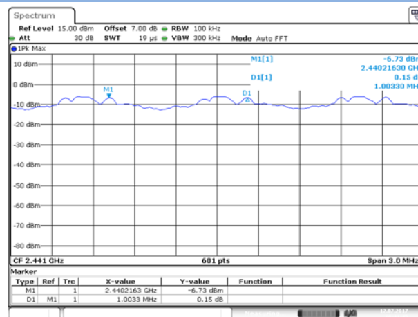
\Pi/4 -DQPSK
