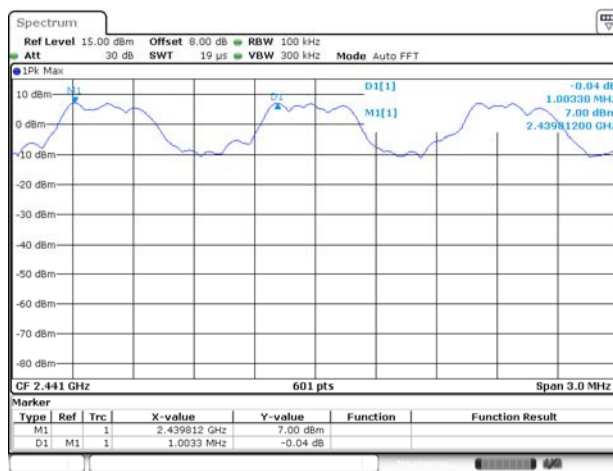
GFSK
