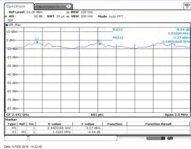
\Pi/4 -DQPSK
