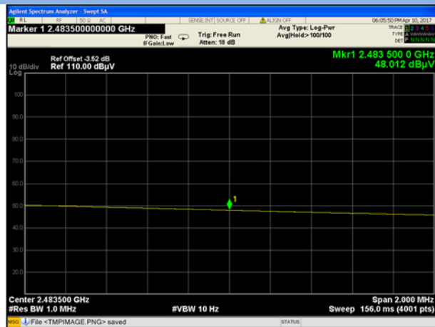
GFSK HIGH CHANNEL , AV
