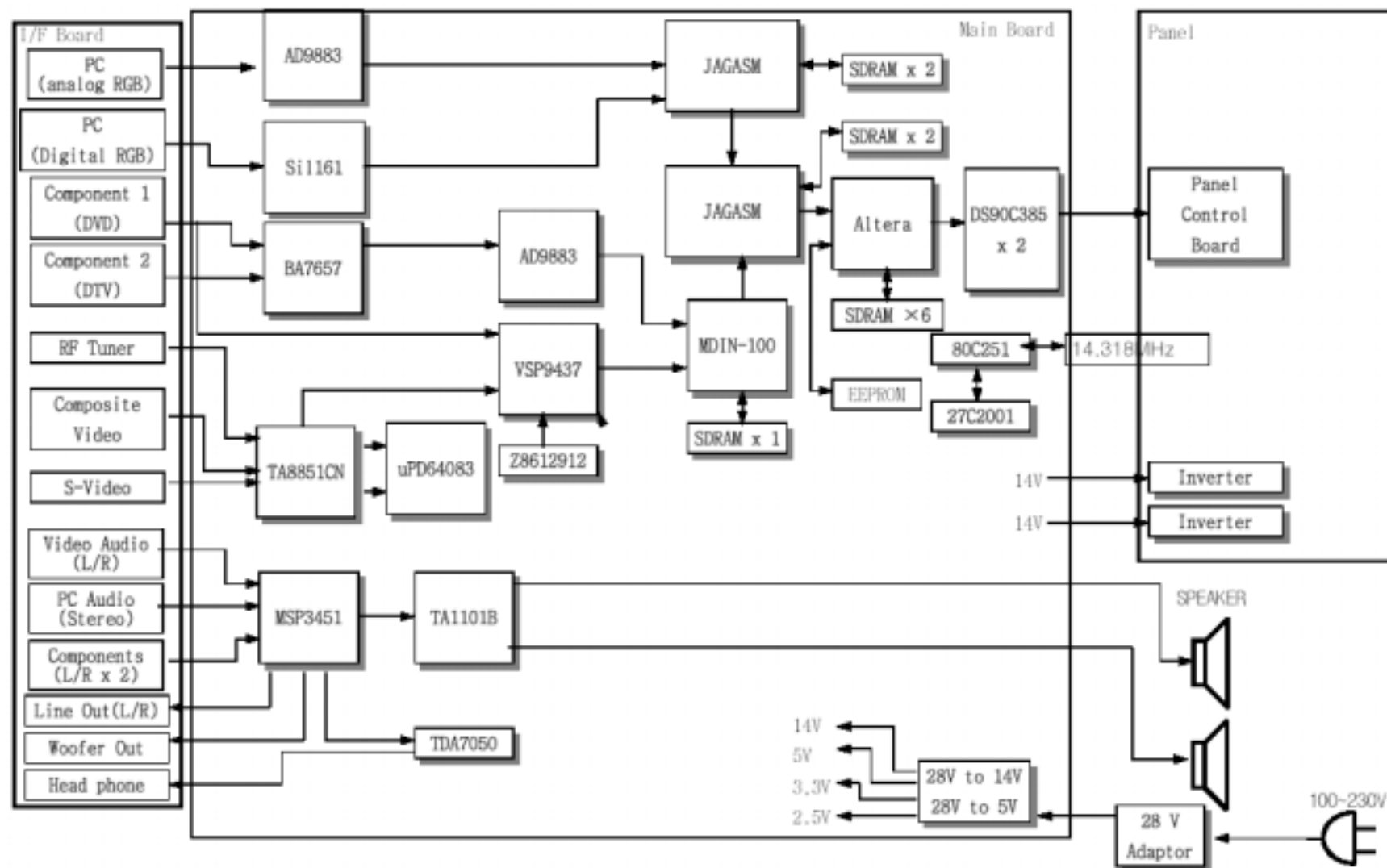
AL40NO/AN29NO Block diagram(NTSC)
