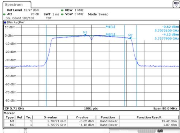
802.11n HT40
