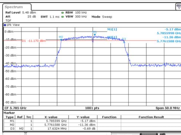
UNII-3 / 802.11ac VHT 20 / Mid ch.
