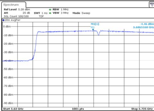
UNII-2C / 802.11ac VHT80
