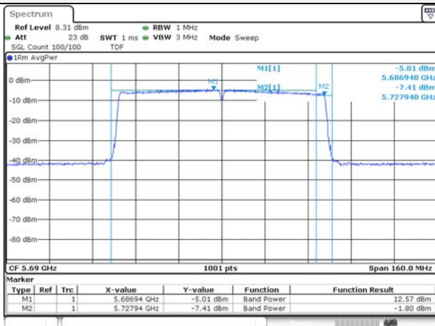
802.11ac VHT80
