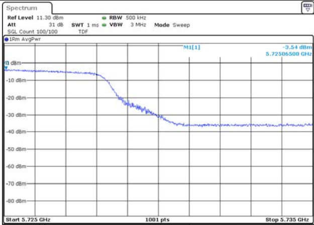
UNII-3 / 802.11a
