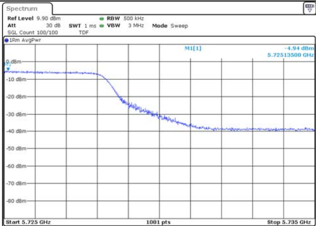
UNII-3 / 802.11n HT40
