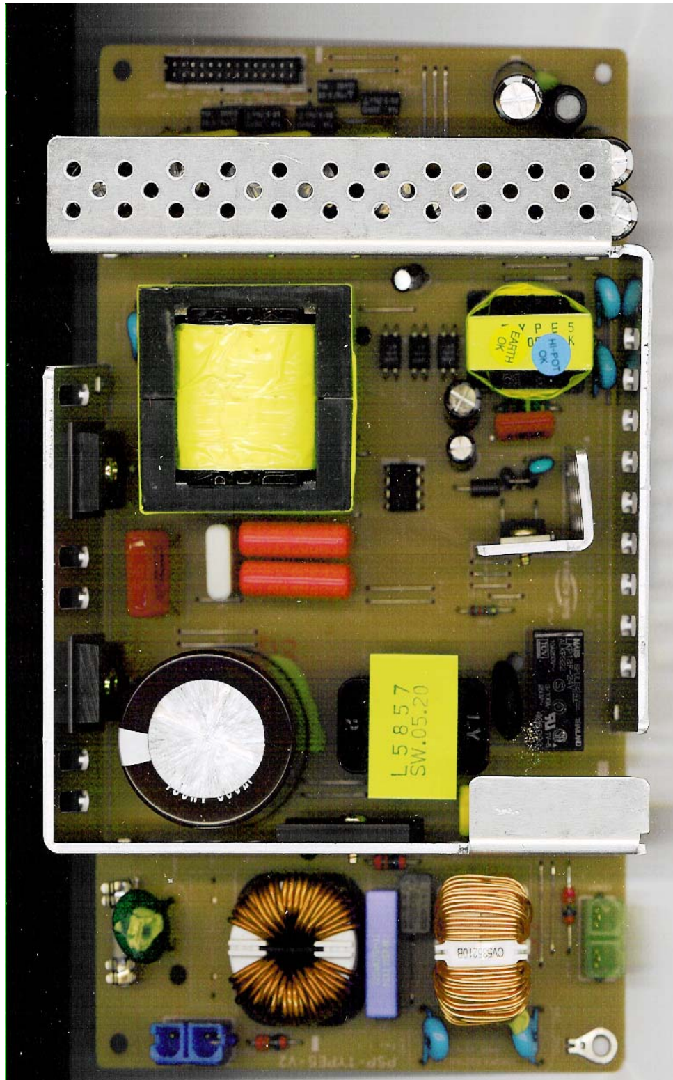
Fig. 03 SMPS PBA
