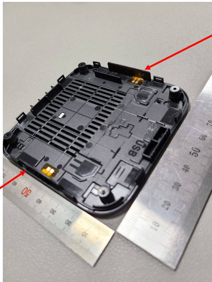
BT/WiFi Antenna
