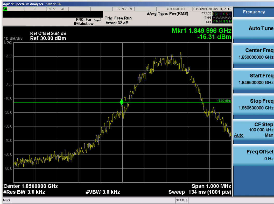
Plot 8-3. Band Edge Plot (PCS GSM Mode (Aux. Ant.) – Ch. 512)
