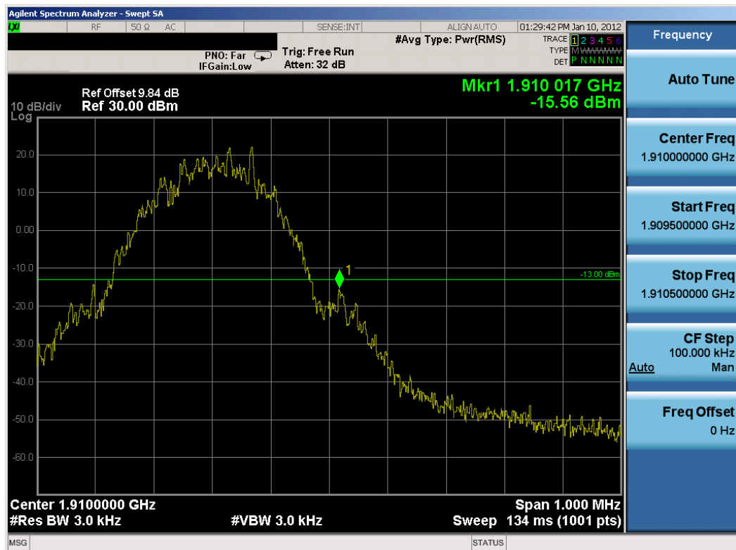
Plot 8-10. Band Edge Plot (PCS GSM Mode (Aux. Ant.) – Ch. 810)
