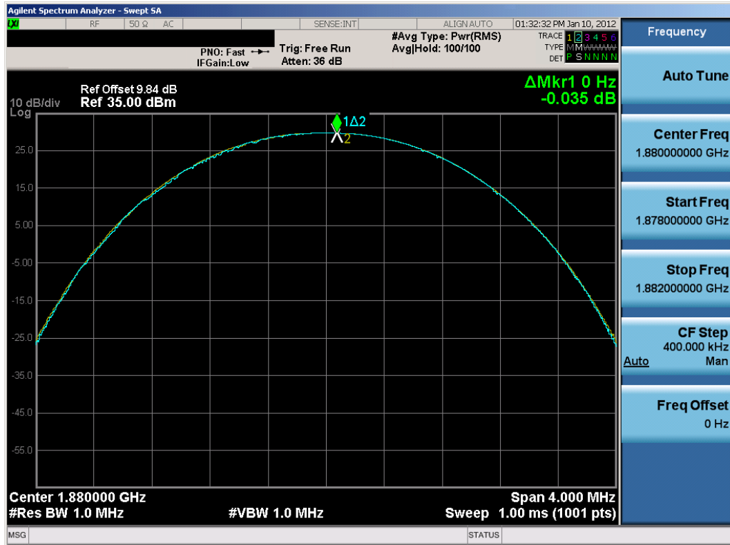
Plot 8-7. Peak-Average Ratio Plot (PCS GSM Mode (Aux. Ant.) - Ch. 661)
