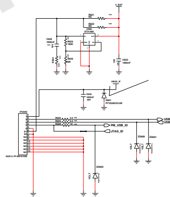
USB CON WITH FET
