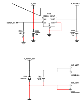
DC MOTOR
