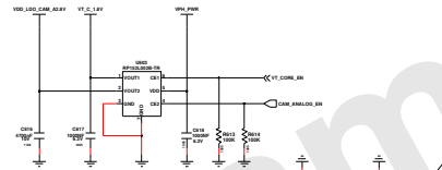
CAM LDO
