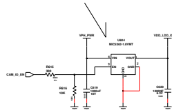
CAM IO LDO
