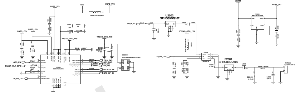
GPS ANT
