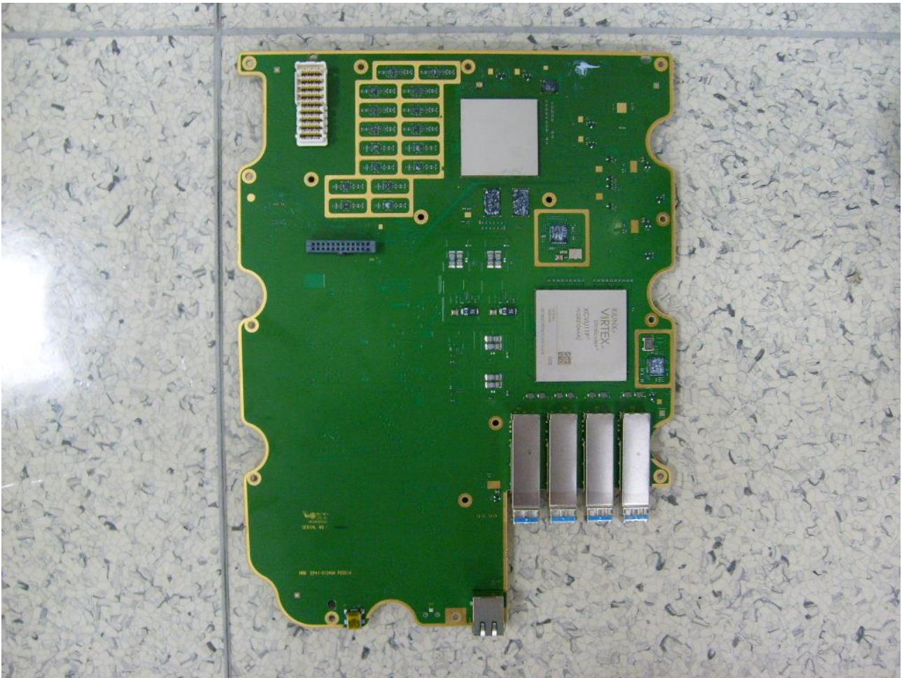
[HRB Module_Top]
