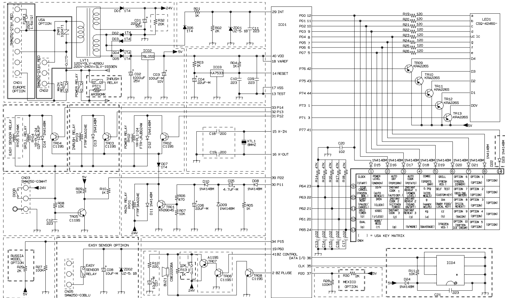
N2LED1 SCHEMATIC
