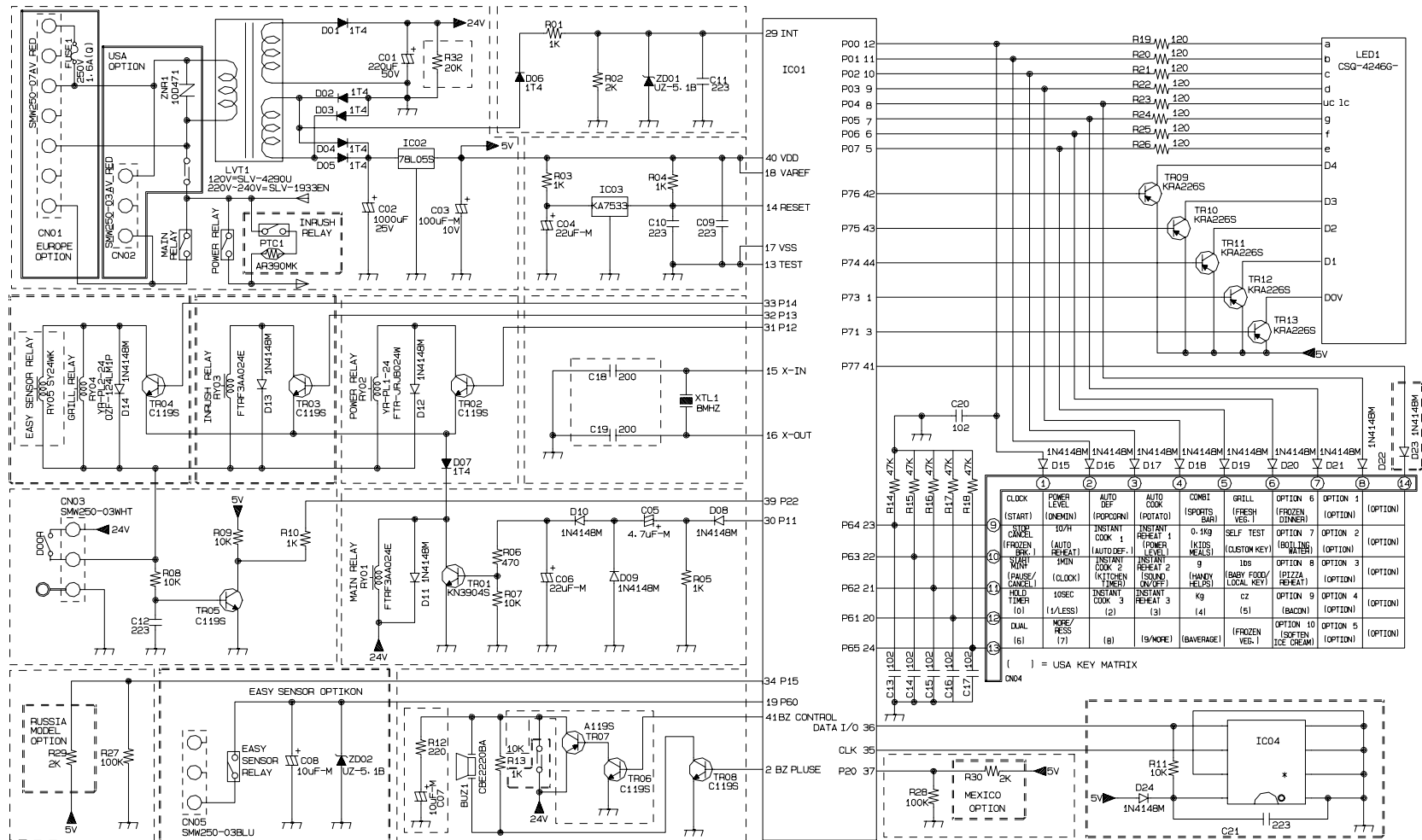
N2LED1 SCHEMATIC
