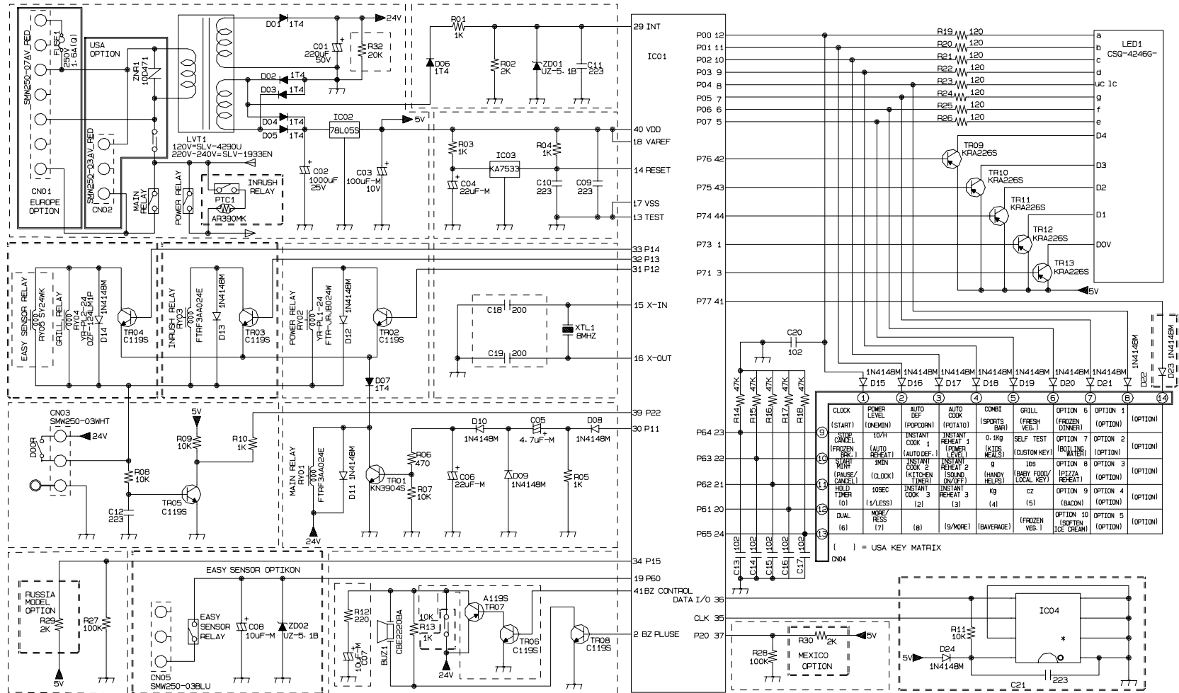
N2LED1 SCHEMATIC
