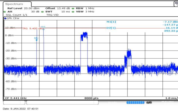
3DH1_Ant1_Hop
