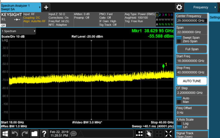
18 GHz ~ 40 GHz Aver
