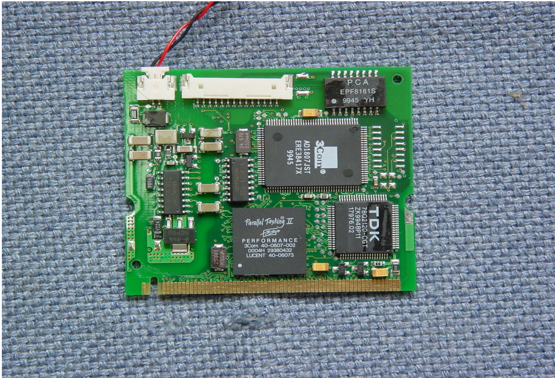
Rear side of Mini PCI
