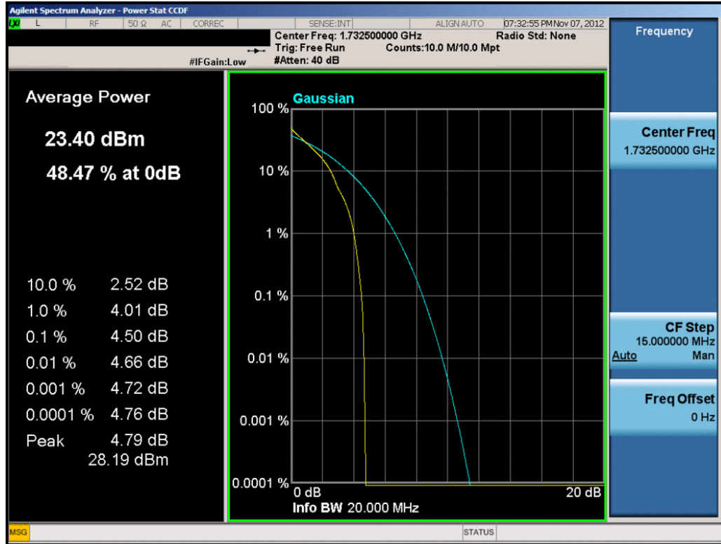
Plot 8-55. PAR Plot (20.0MHz QPSK – RB Size 100)
