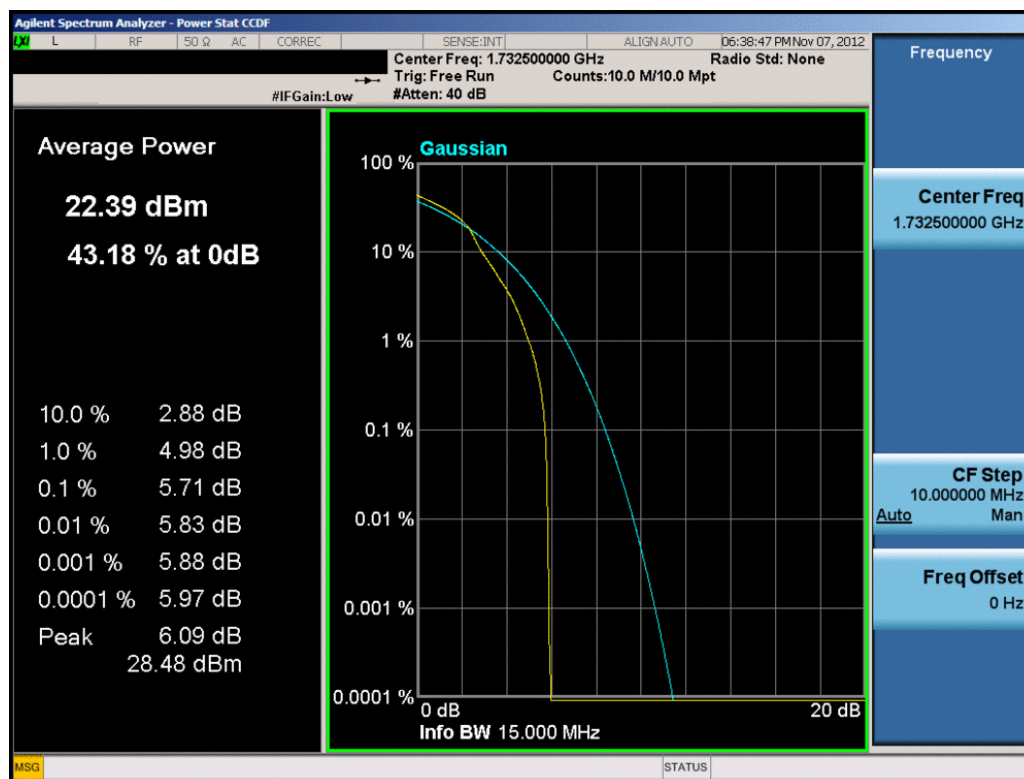
Plot 8-42. PAR Plot (15.0MHz 16-QAM – RB Size 75)
