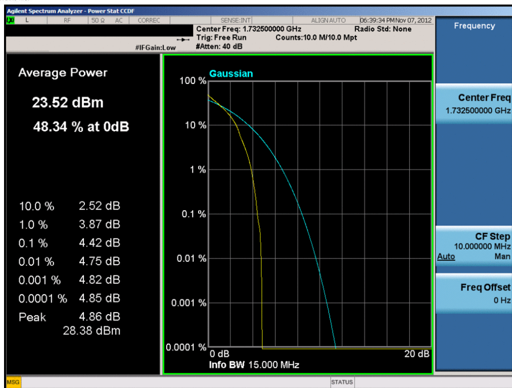
Plot 8-41. PAR Plot (15.0MHz QPSK – RB Size 75)
