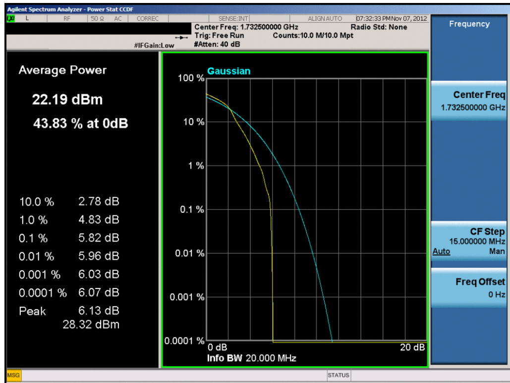
Plot 8-56. PAR Plot (20.0MHz 16-QAM – RB Size 100)
