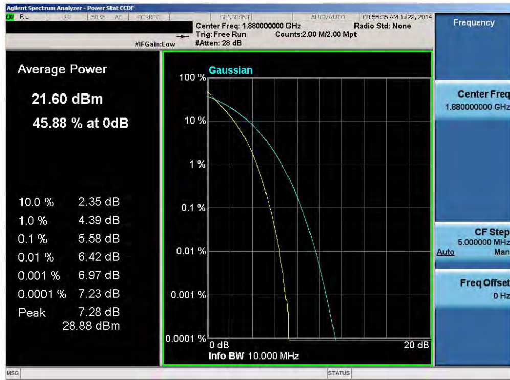
Plot 6-61. PAR Plot (Band 2 – 10.0MHz QPSK – RB Size 50)
