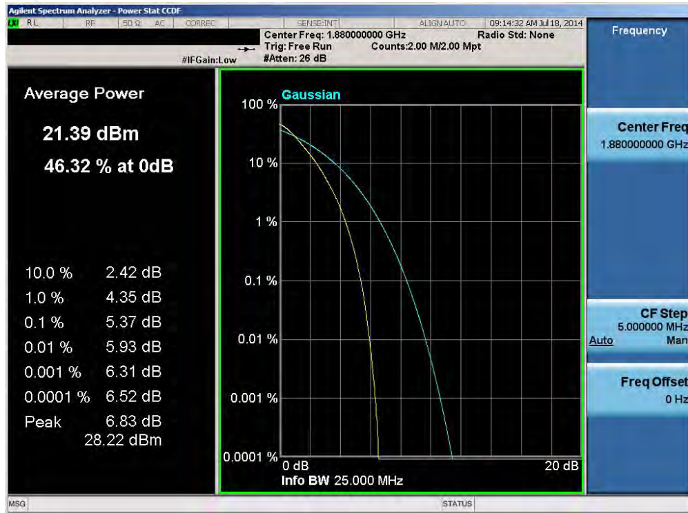
Plot 6-65. PAR Plot (Band 2 – 20.0MHz QPSK – RB Size 100)
