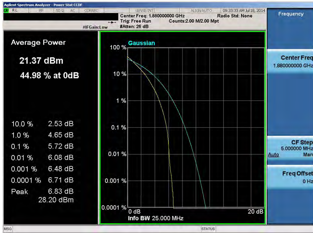
Plot 6-63. PAR Plot (Band 2 – 15.0MHz QPSK – RB Size 75)
