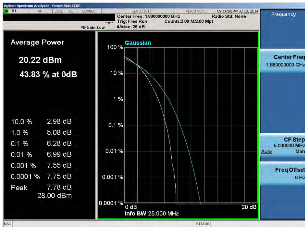
Plot 6-66. PAR Plot (Band 2 – 20.0MHz 16-QAM – RB Size 100)
