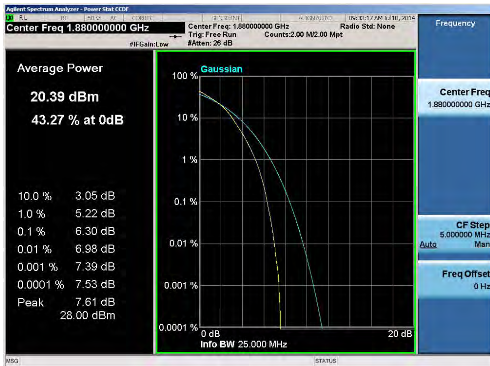
Plot 6-64. PAR Plot (Band 2 – 15.0MHz 16-QAM – RB Size 75)
