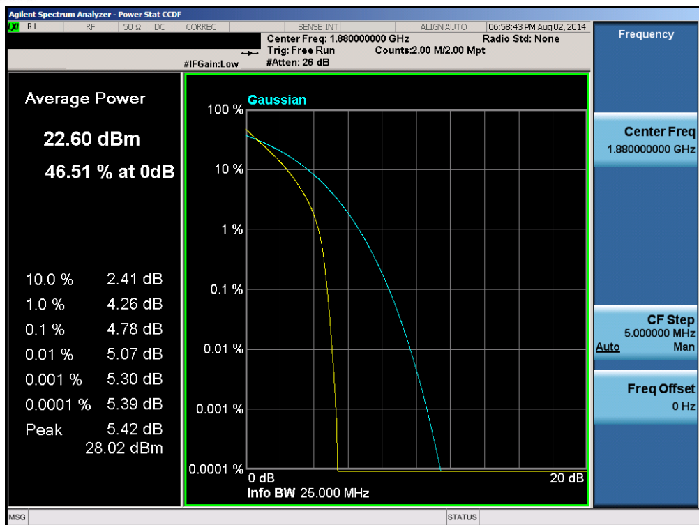
Plot 6-27. PAR Plot (Band 2 – 20.0MHz QPSK – RB Size 100)
