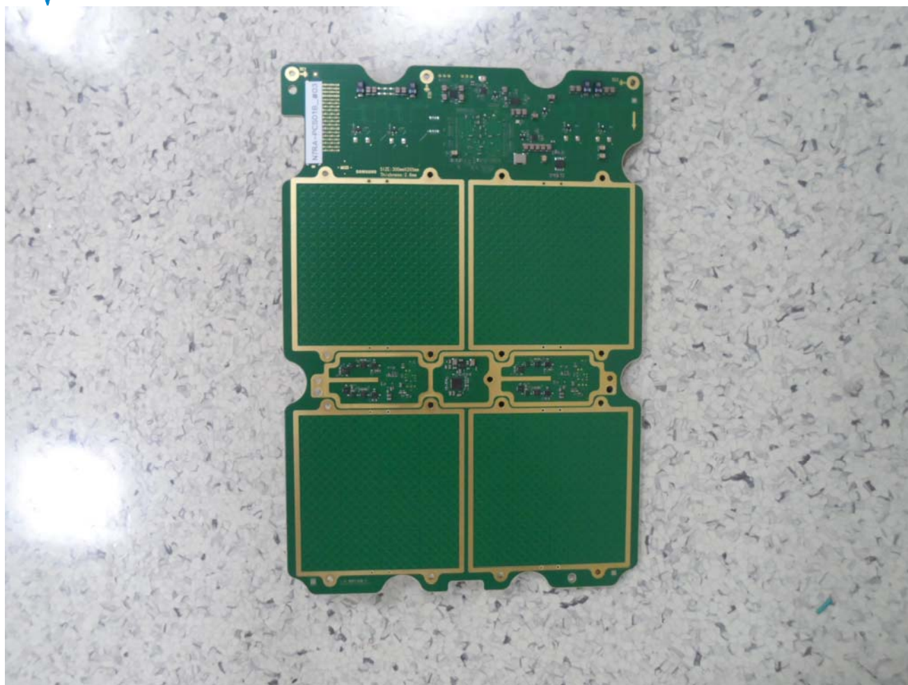
N7RA Module (Bottom)
