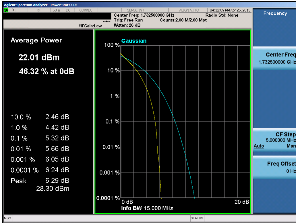
Plot 9-23. PAR Plot (15.0MHz QPSK – RB Size 75)
