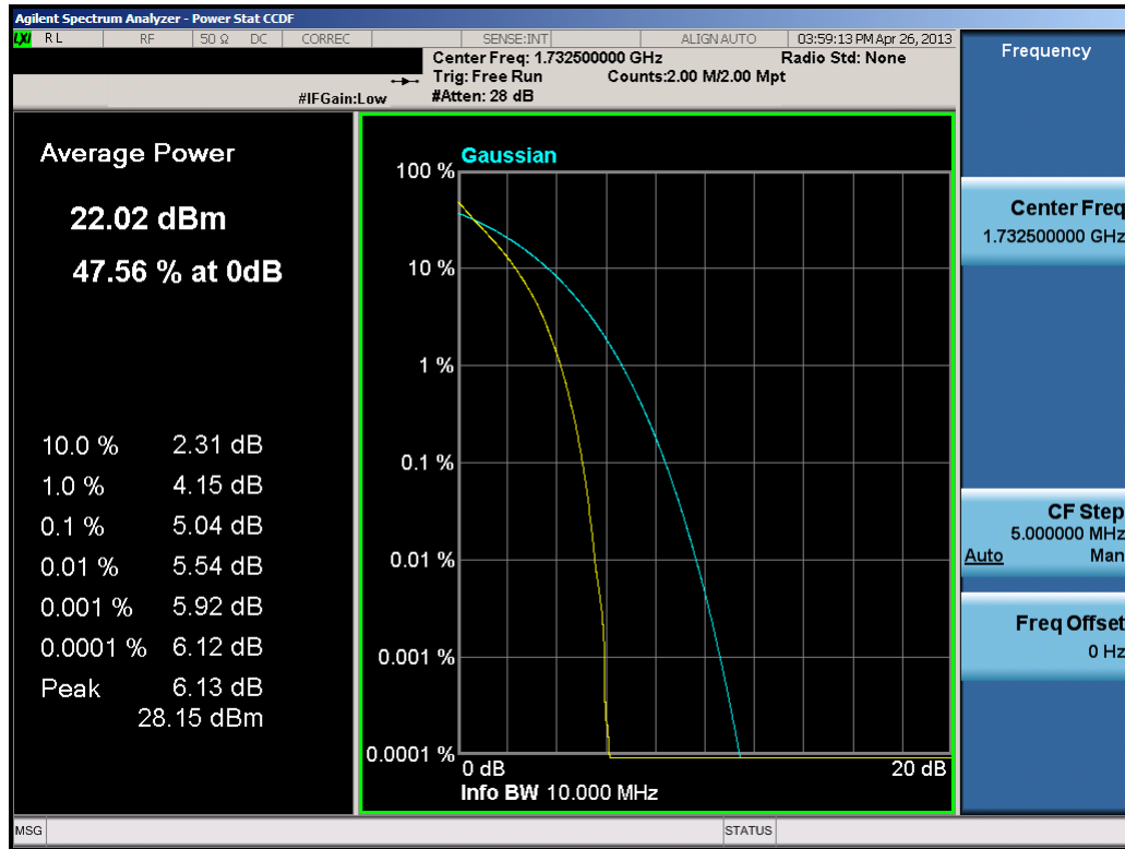
Plot 9-15. PAR Plot (10.0MHz QPSK – RB Size 50)
