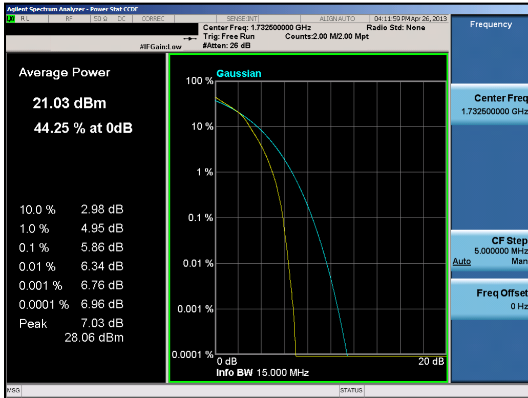
Plot 9-24. PAR Plot (15.0MHz 16-QAM – RB Size 75)
