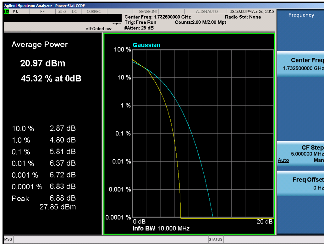
Plot 9-16. PAR Plot (10.0MHz 16-QAM – RB Size 50)
