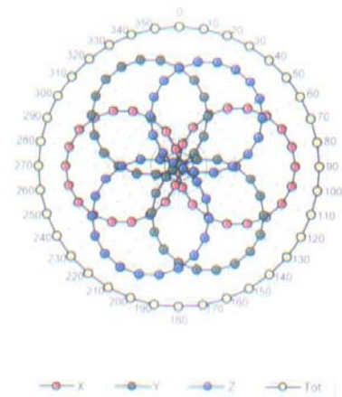
f = 600 MHz, TEM ifi110EXX
