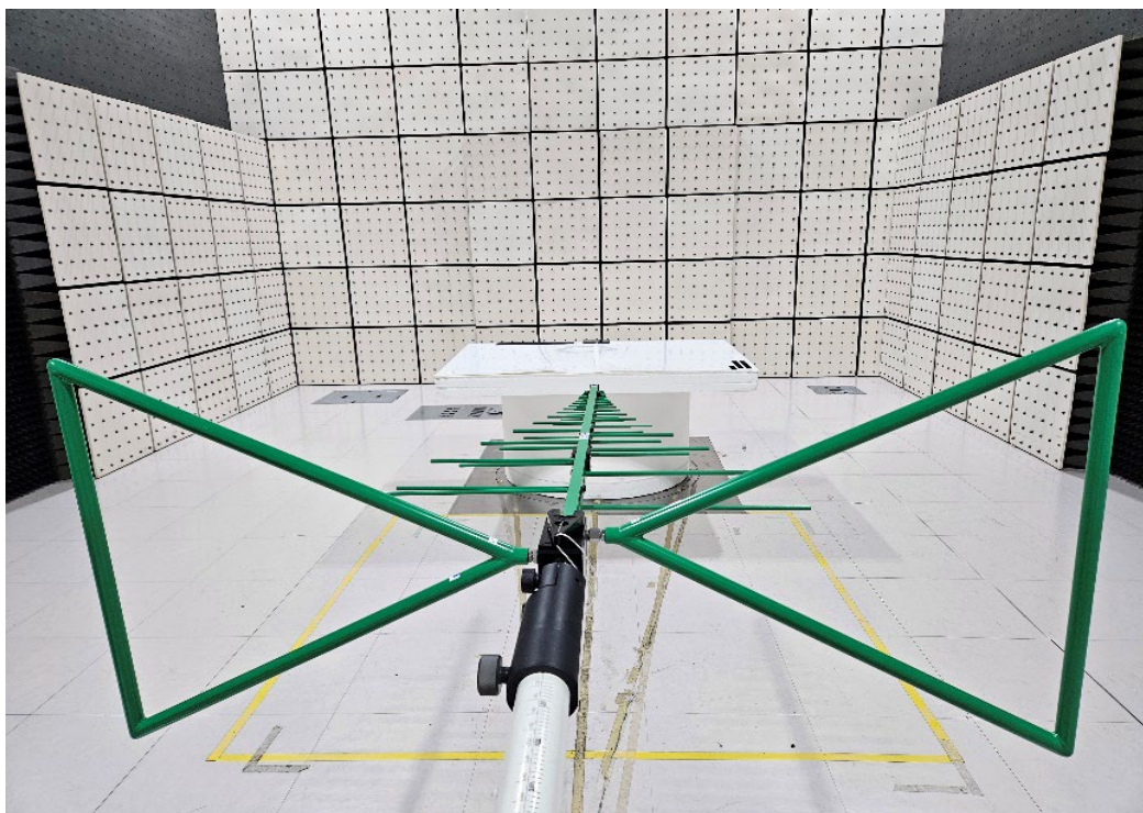
- Mode 3
