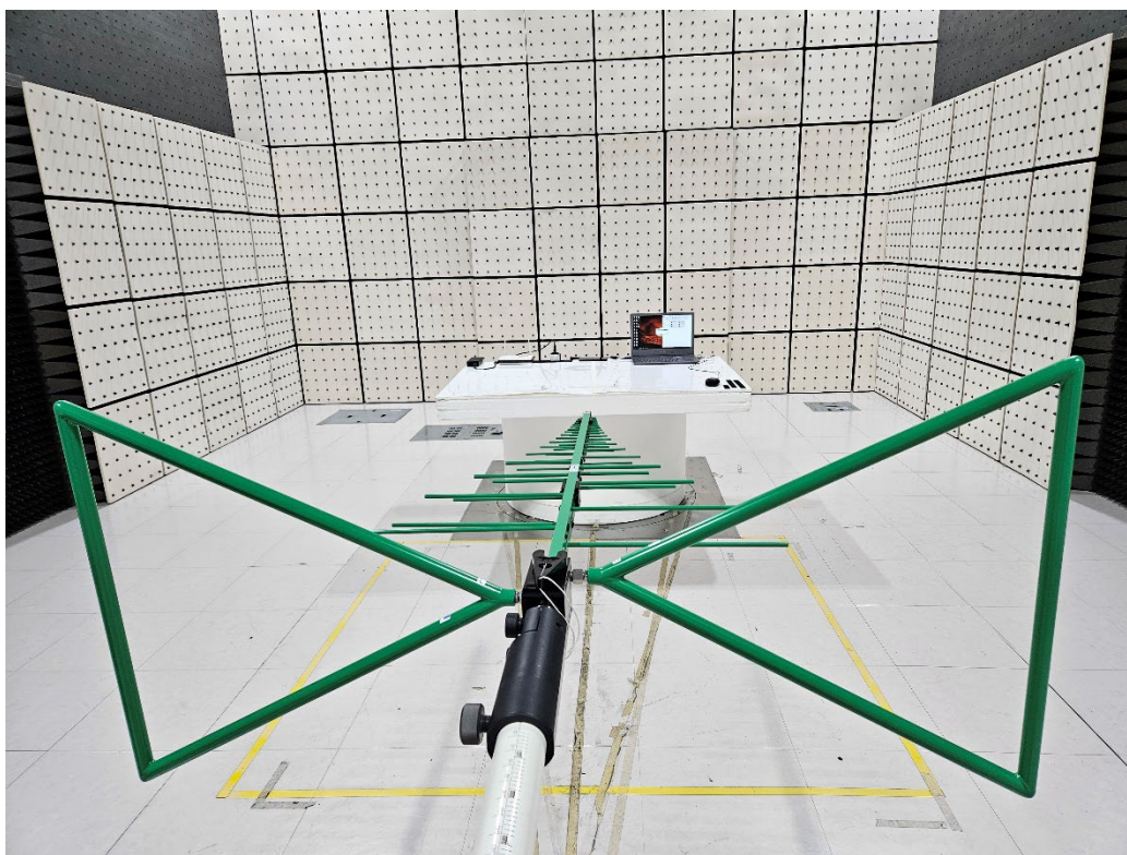
- Mode 4
