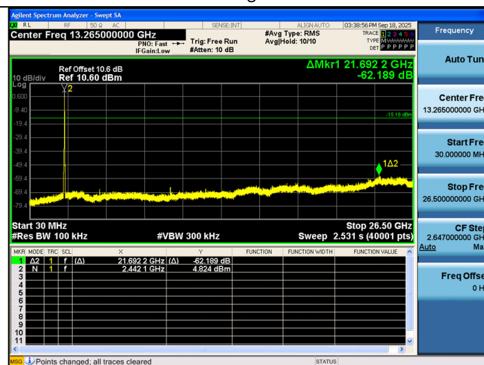
802.11g - CH 6
