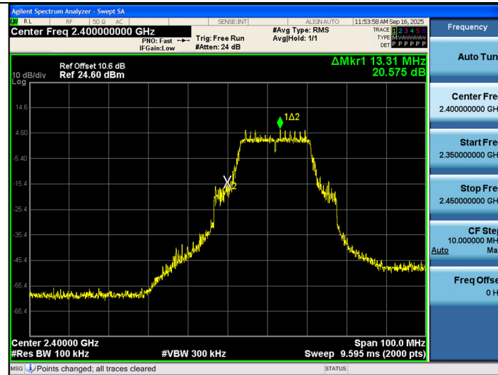
802.11n(HT20) - CH 1
