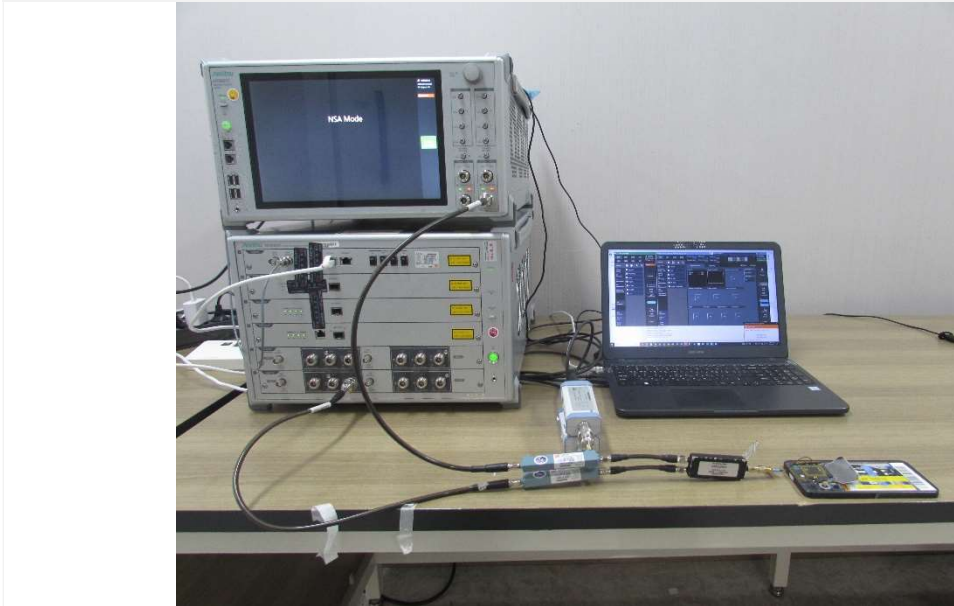
Test setup photo-5 TC13
