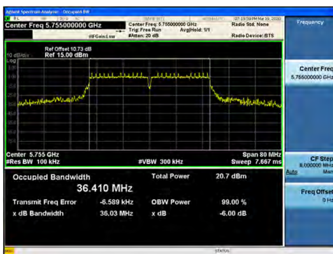
802.11ac(VHT40) (CH.151)
