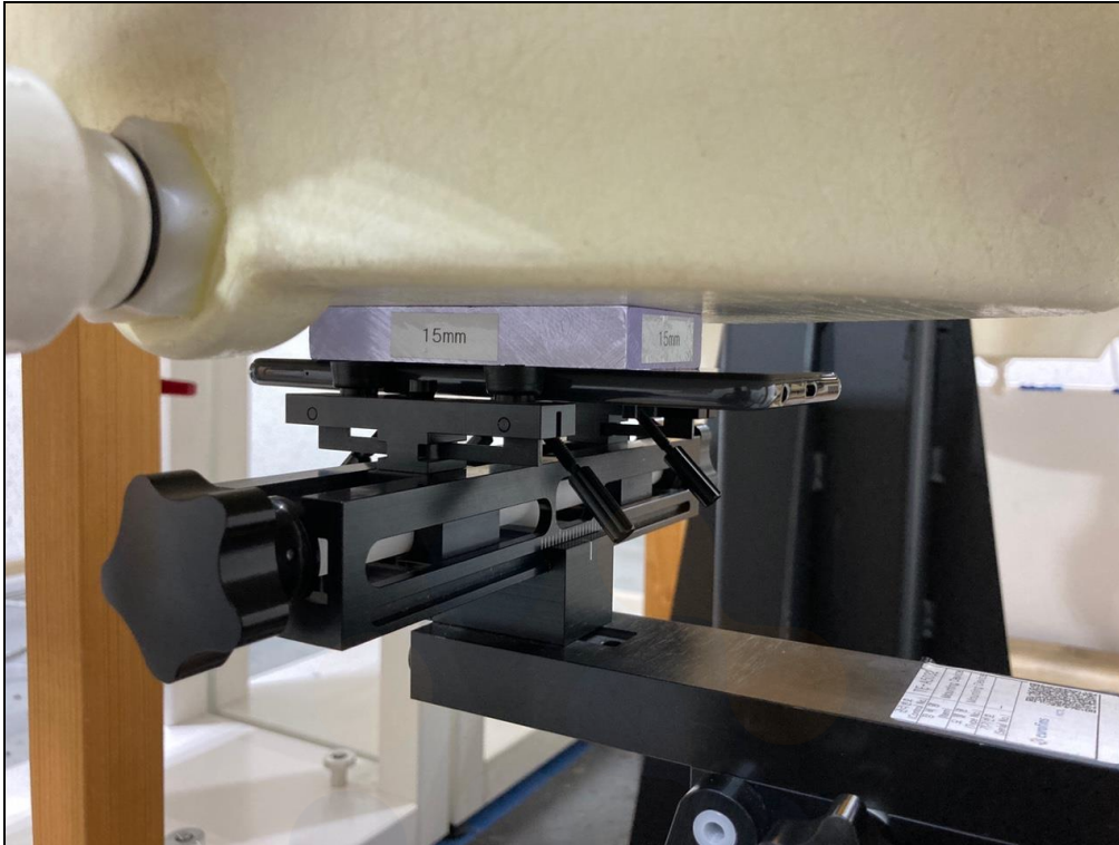
F.2.1) Body-Worn_Front (15mm)
