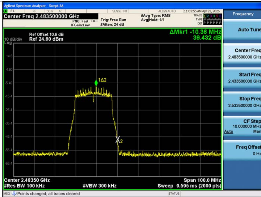
802.11ac(VHT20)- CH 13
