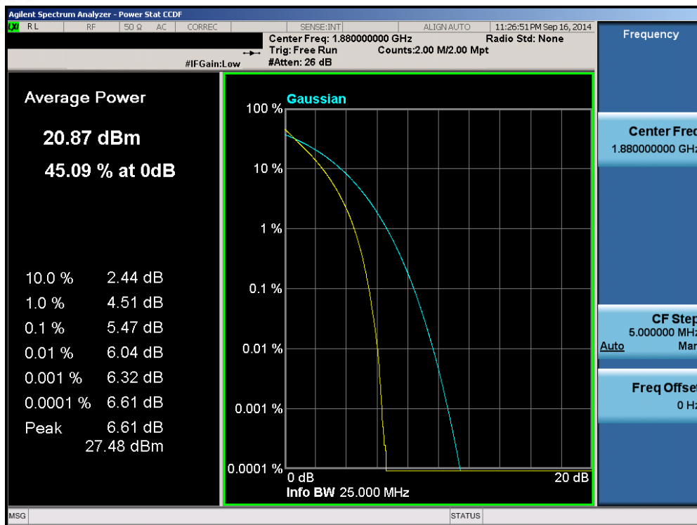
Plot 6-131. PAR Plot (Band 2 – 20.0MHz QPSK – RB Size 100)
