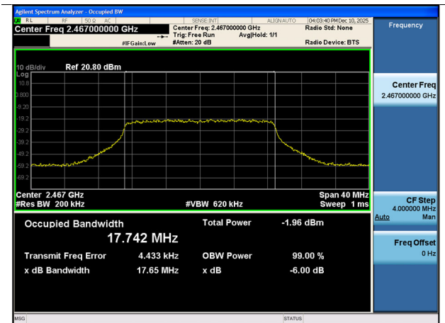
802.11n_HT20-CH 12
