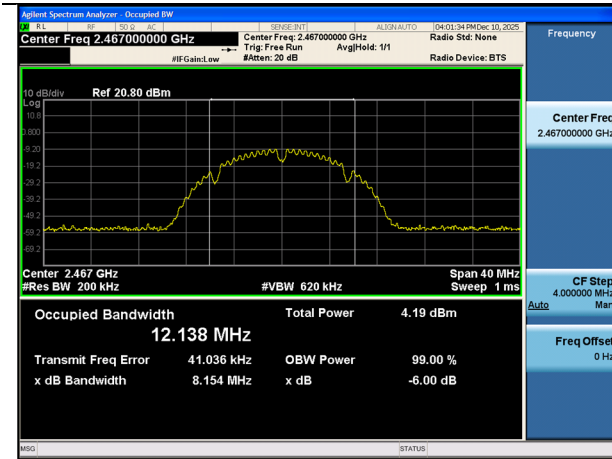
802.11n_HT20-CH 12
