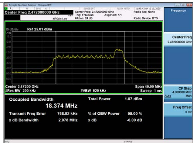
BW20M Ch.13(2472 MHz) RU 8
