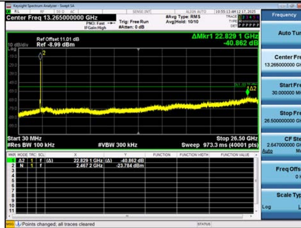
[MIMO_SDM(Ant.1)] BW 20M Ch.12(2 467 MHz) SU
