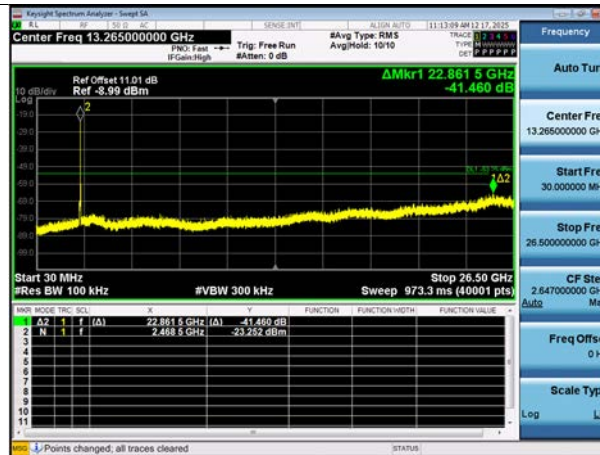
[MIMO_SDM(Ant.2)] BW 20M Ch.13(2 472 MHz) 242T RU 61
