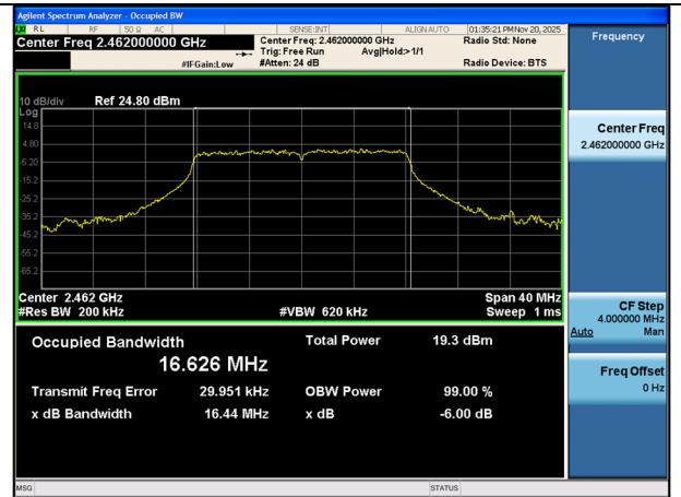
802.11g-CH 11
