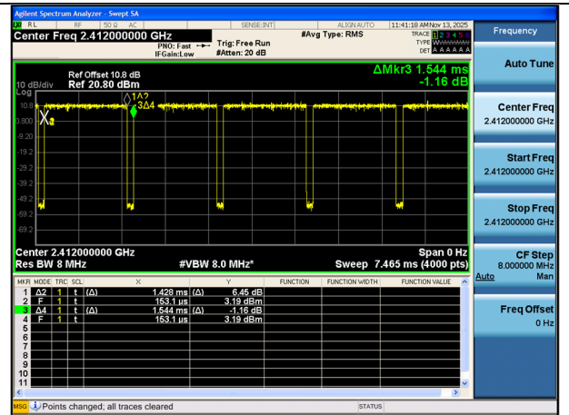
802.11n (MCS8)
