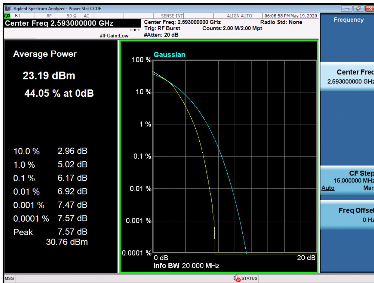
PAR Plot (20M BW_Ch.40620_16QAM_RB100_0) (POWER CLASS 2)
