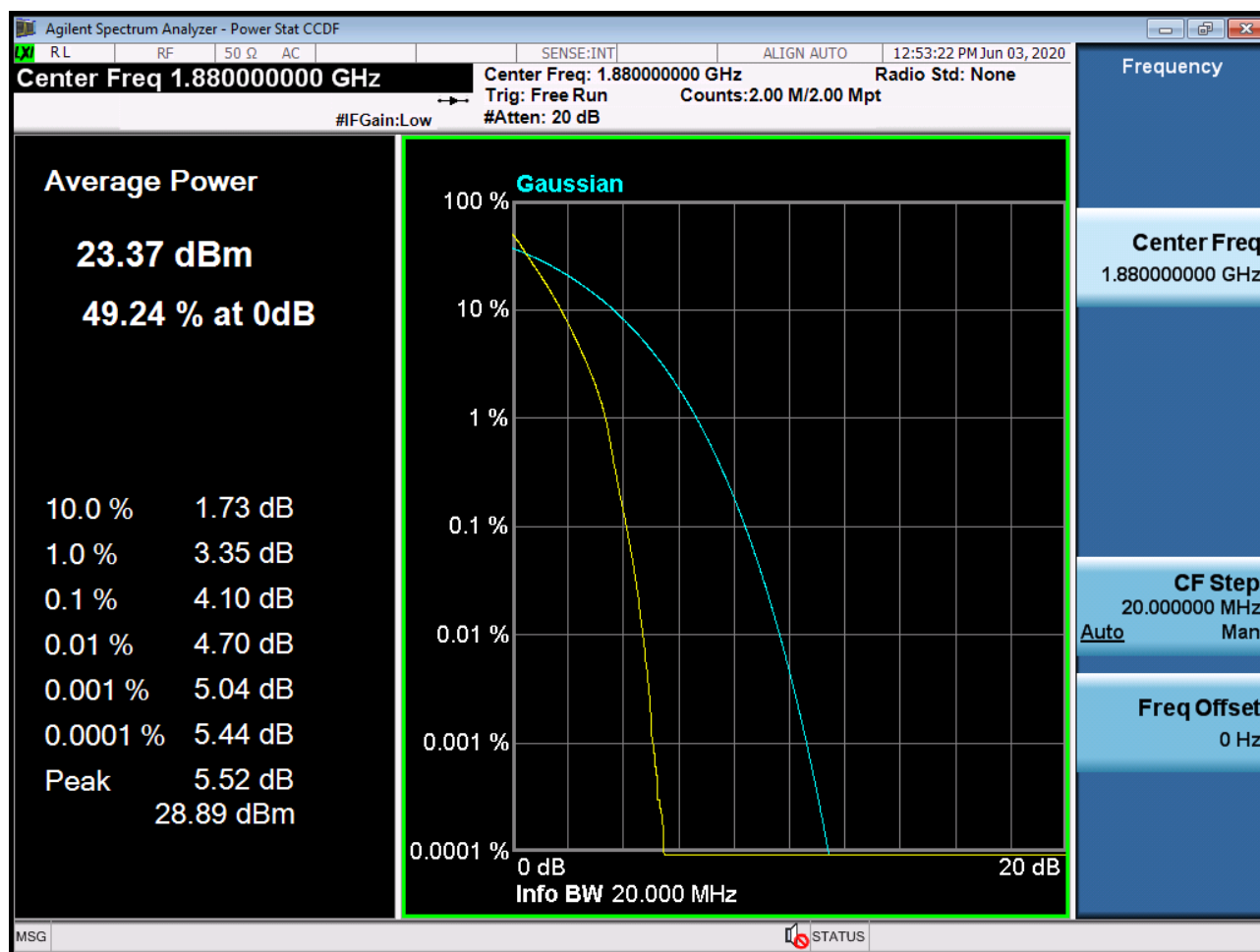
Sub6 n2. PAR Plot (20M BW Ch.376000 BPSK RB 100_0)
