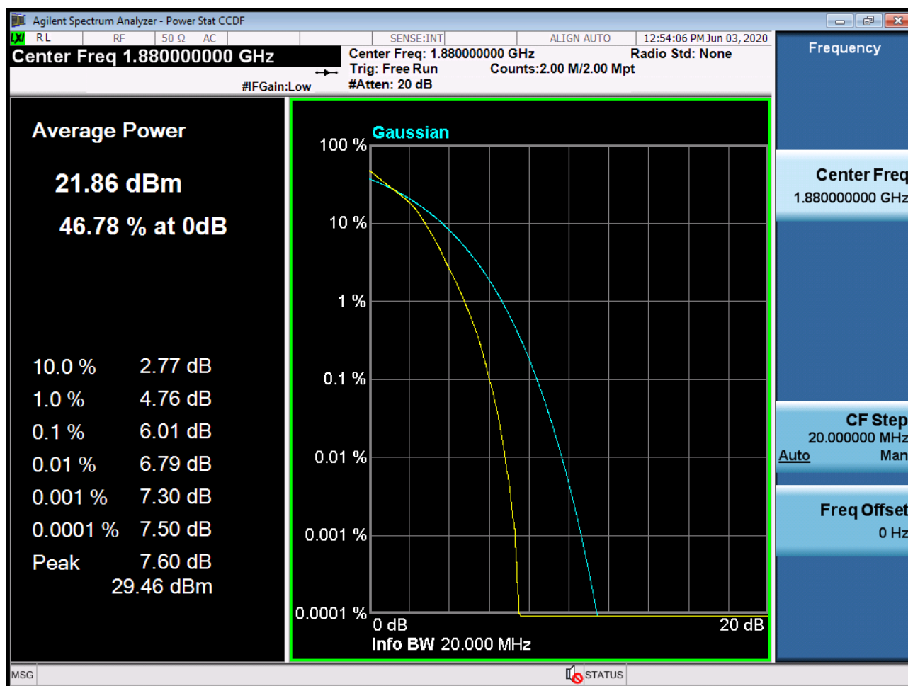
Sub6 n2. PAR Plot (20M BW Ch.376000 16QAM RB 100_0)
