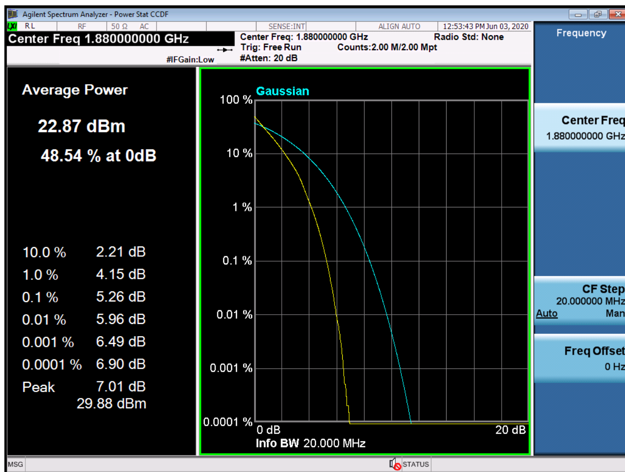
Sub6 n2. PAR Plot (20M BW Ch.376000 QPSK RB 100_0)
