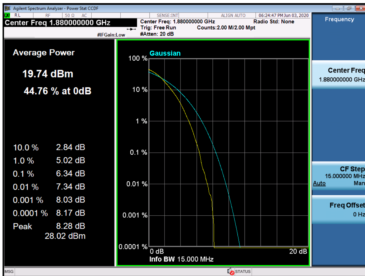
Sub6 n2. PAR Plot (15M BW Ch.376000 256QAM RB 75_0)
