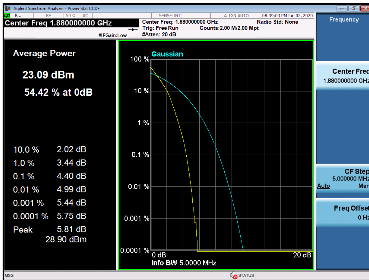
Sub6 n2. PAR Plot (5M BW Ch.376000 BPSK RB 25_0)
