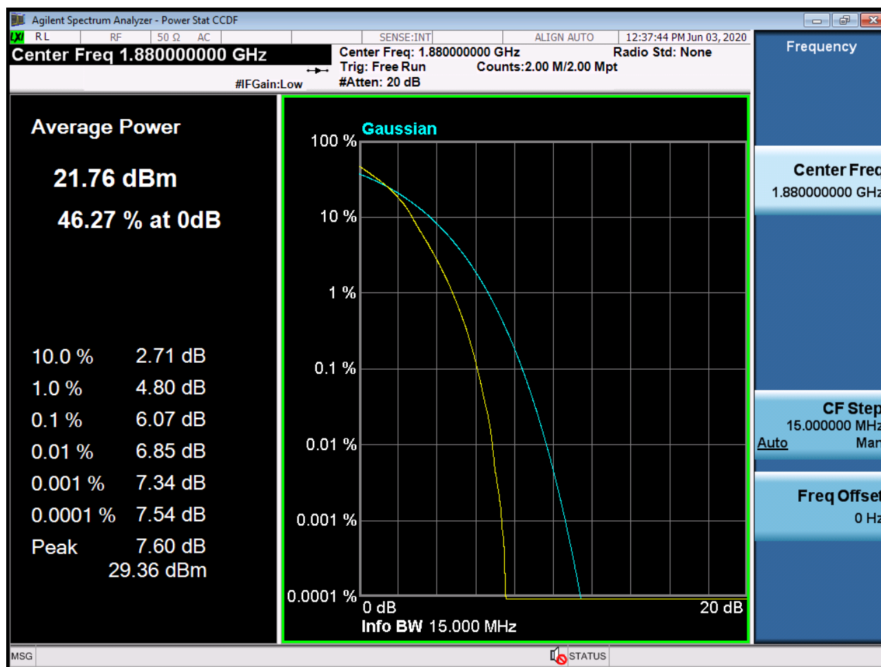
Sub6 n2. PAR Plot (15M BW Ch.376000 16QAM RB 75_0)
