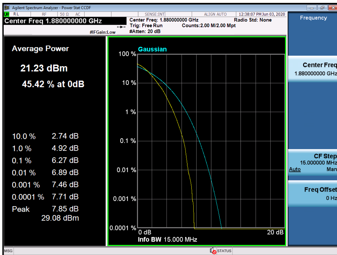
Sub6 n2. PAR Plot (15M BW Ch.376000 64QAM RB 75_0)
