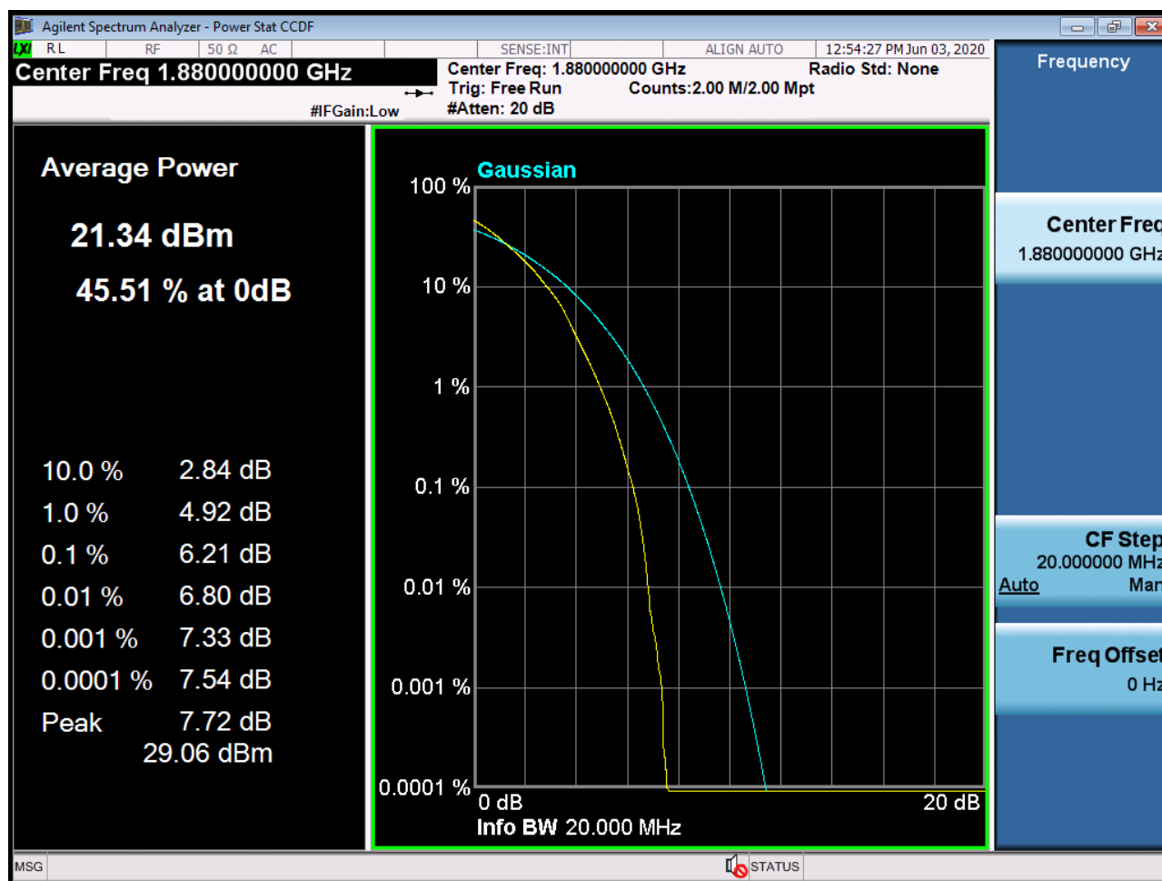
Sub6 n2. PAR Plot (20M BW Ch.376000 64QAM RB 100_0)
