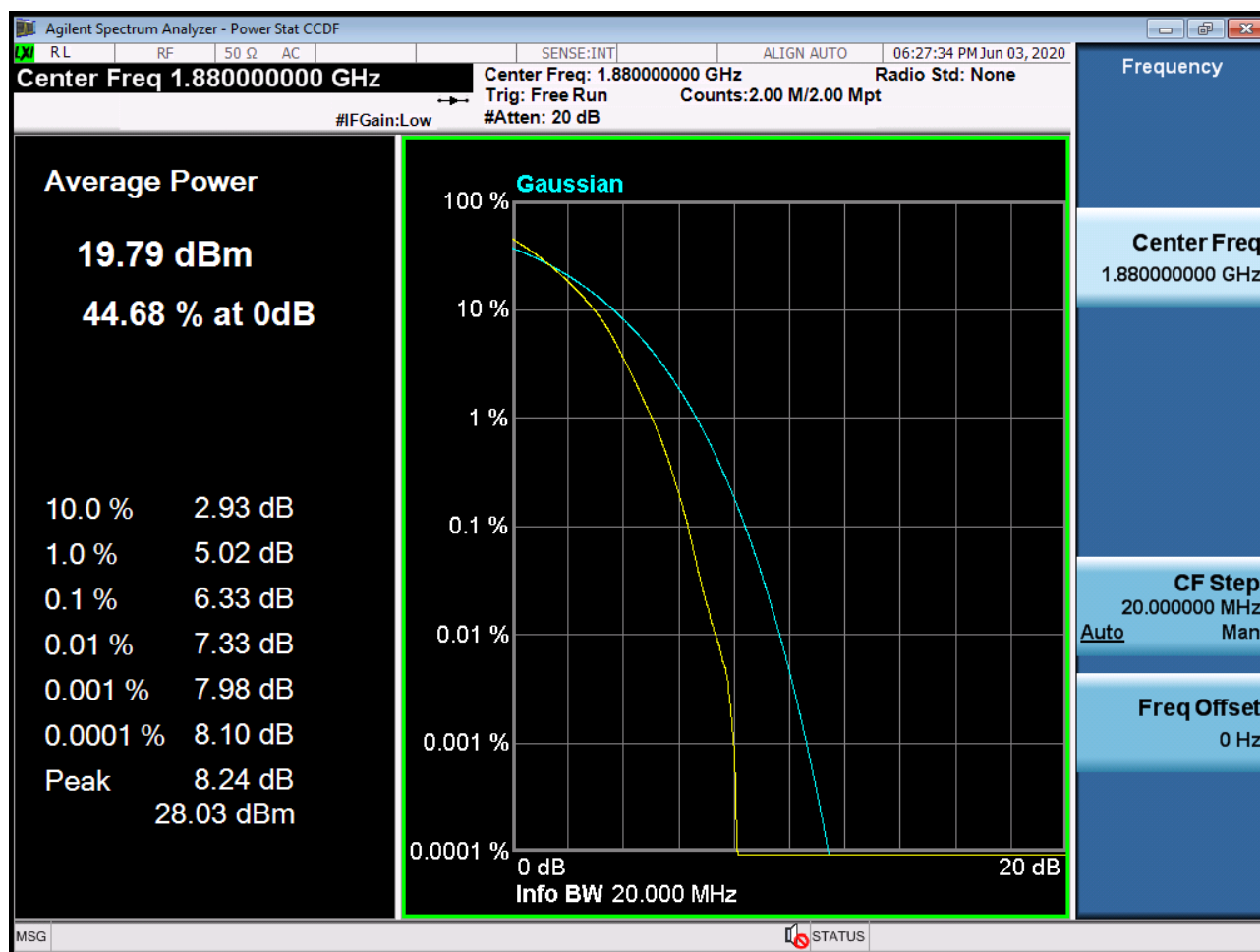
Sub6 n2. PAR Plot (20M BW Ch.376000 256QAM RB 100_0)
