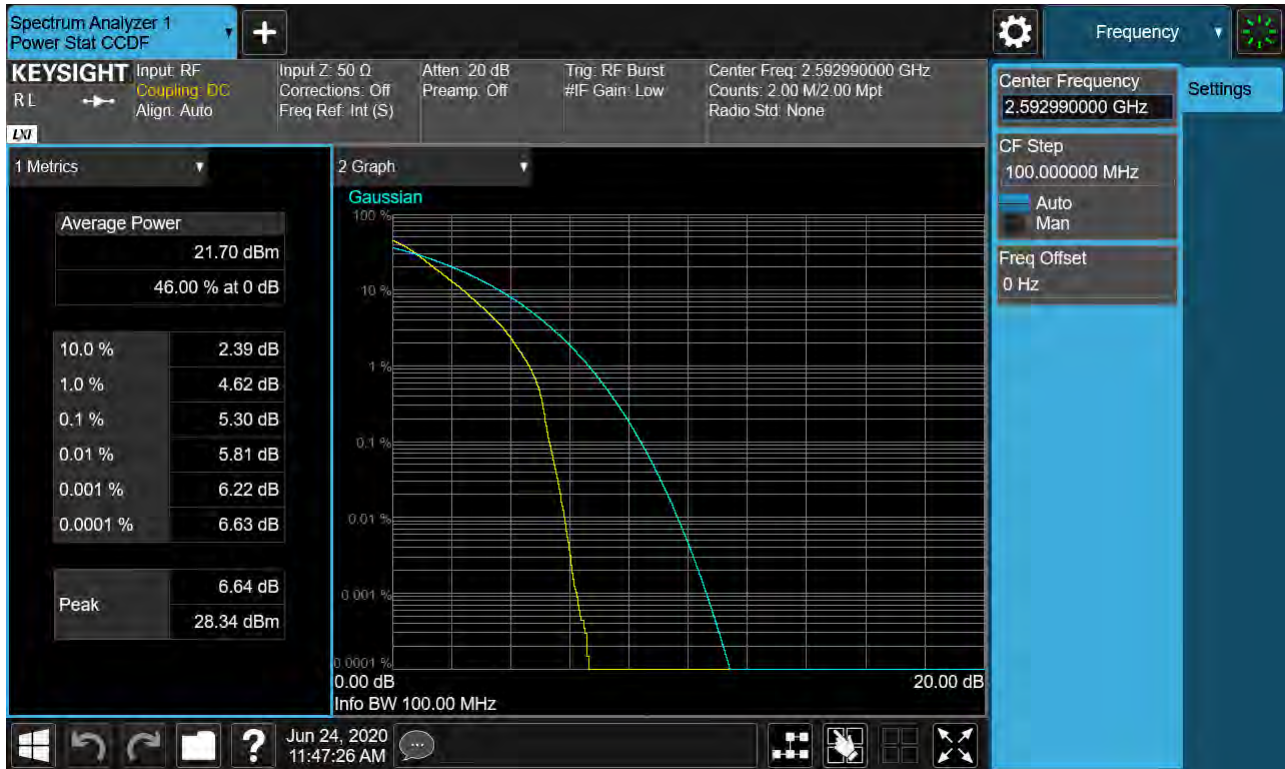
Sub6 n41. PAR Plot (100M BW_Ch.518598_QPSK_RB25_0)
