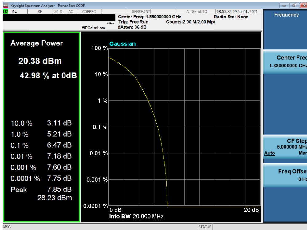
Plot 7-74. PAR Plot (LTE Band 2 - 20MHz 64-QAM - Full RB)
