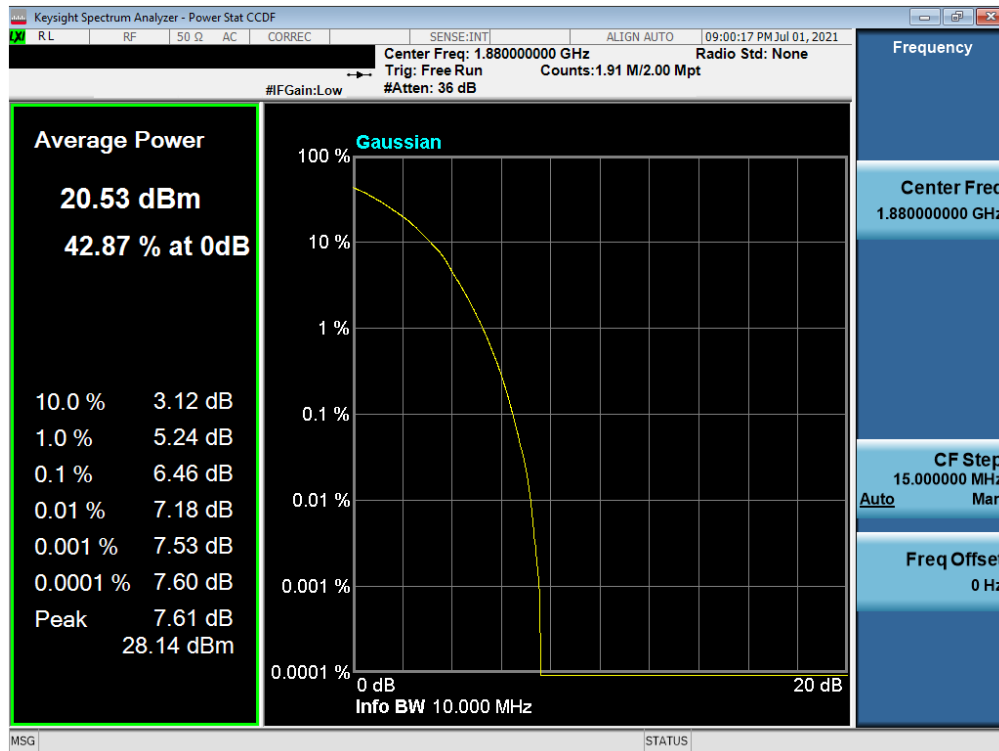
Plot 7-78. PAR Plot (LTE Band 2 - 10MHz 64-QAM - Full RB)
