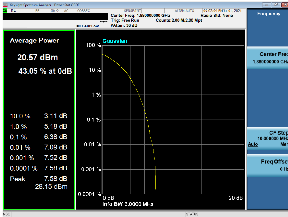
Plot 7-80. PAR Plot (LTE Band 2 - 5MHz 64-QAM - Full RB)
