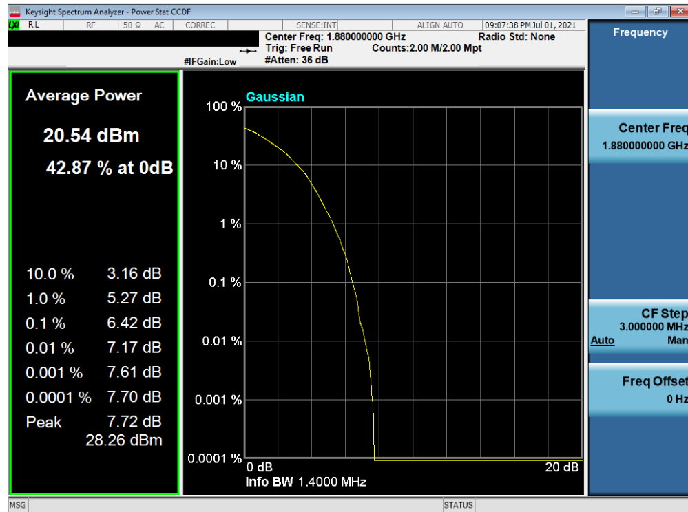
Plot 7-84. PAR Plot (LTE Band 2 - 1.4MHz 64-QAM - Full RB)
