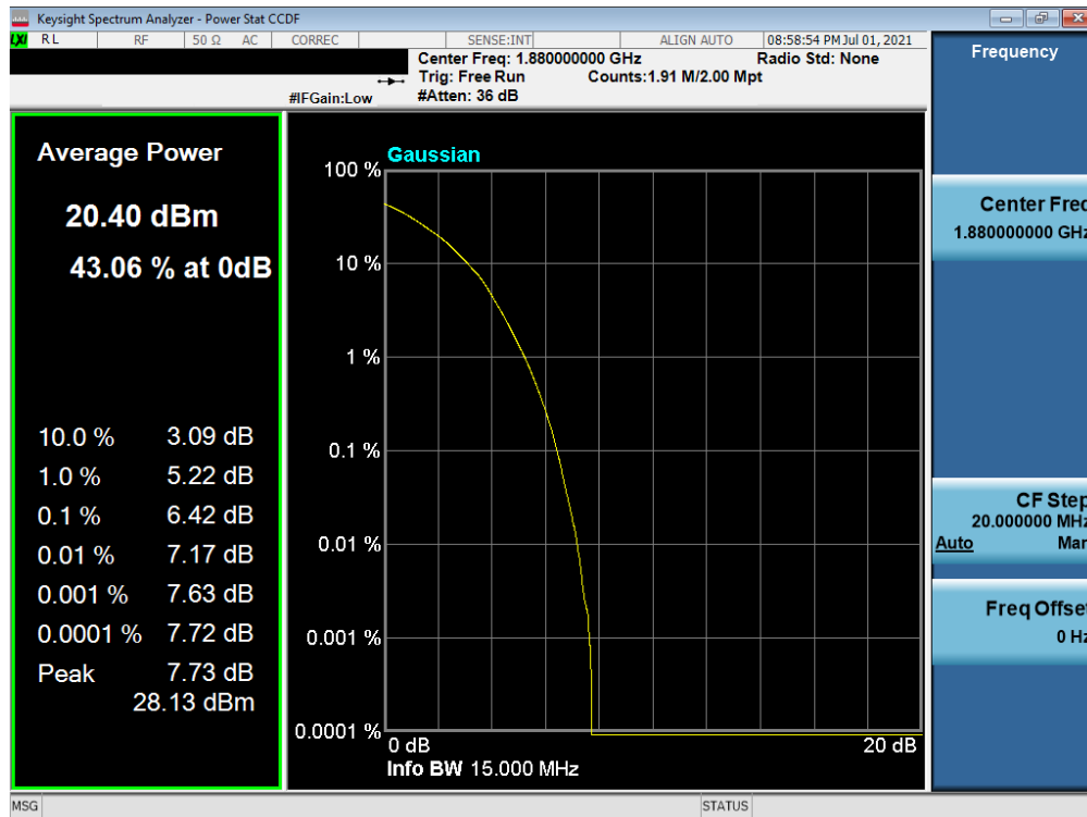
Plot 7-76. PAR Plot (LTE Band 2 - 15MHz 64-QAM - Full RB)
