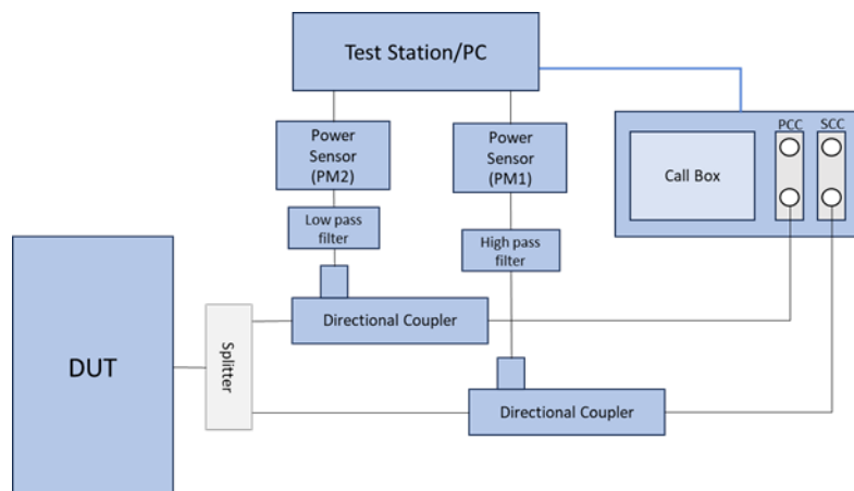
(d) Appendix A – Test Setup Photo 5
