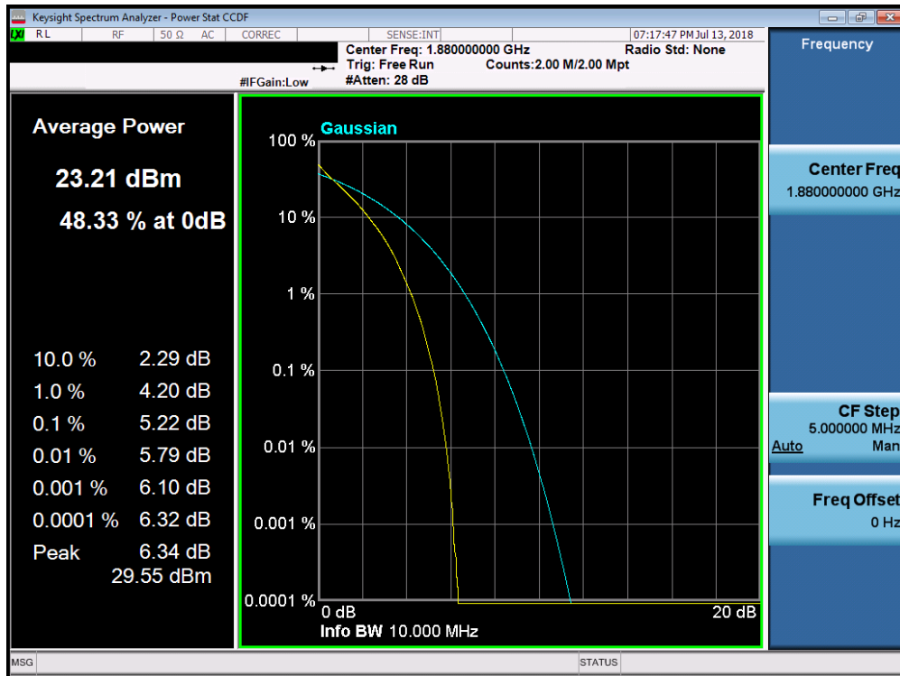
Plot 7-187. PAR Plot (Band 2 - 10.0MHz QPSK - Full RB Configuration)
